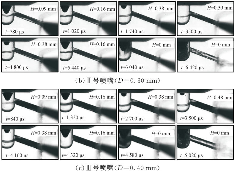
图 9 不同孔径喷嘴内甲醇空化流动的瞬态特性
