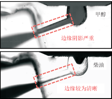
(a)背光成像法下甲醇与柴油瞬态图像对比
