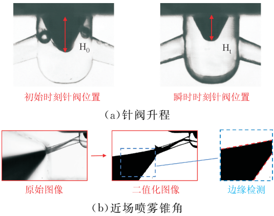
图 5 图像定量处理
