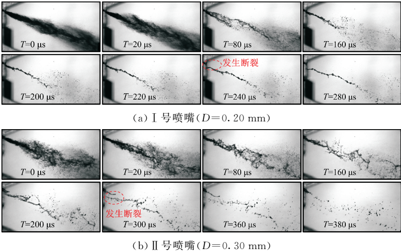
图 10 尾喷阶段不同孔径喷嘴中甲醇近场喷雾瞬态图像
