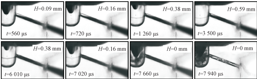
(a) I 号喷嘴( D=0.20 mm)
