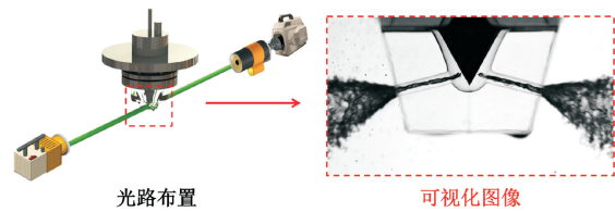
图 3 背光成像法可视化光路布置图
